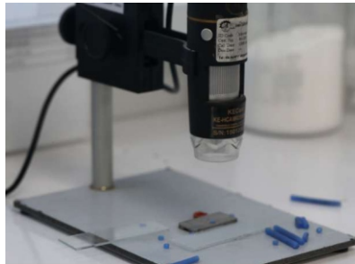
تجهیز میکروسکوپ جهت آزمون ابعادی
